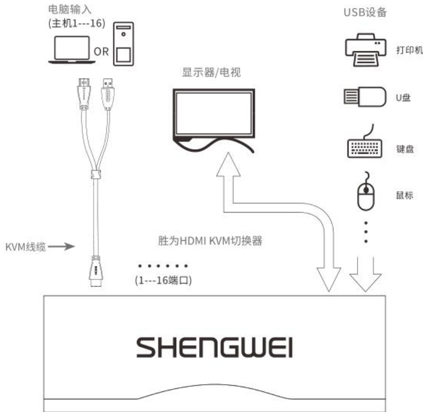
KS-316H安装示意图
